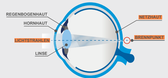
Weitsichtigkeit: Der Brennpunkt liegt hinter der Netzhaut.
