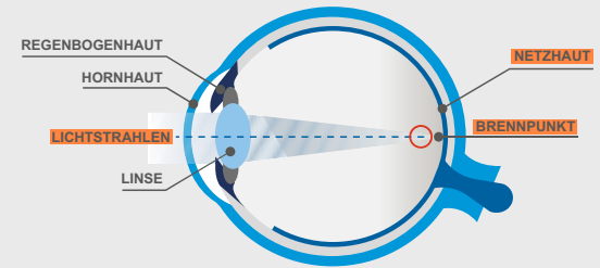
Kurzsichtigkeit: Das Licht trifft vor der Netzhaut auf.
