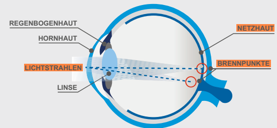
Hornhautverkrümmung: Die Lichtstrahlen treffen an unterschiedlichen Stellen auf der Netzhaut auf.
